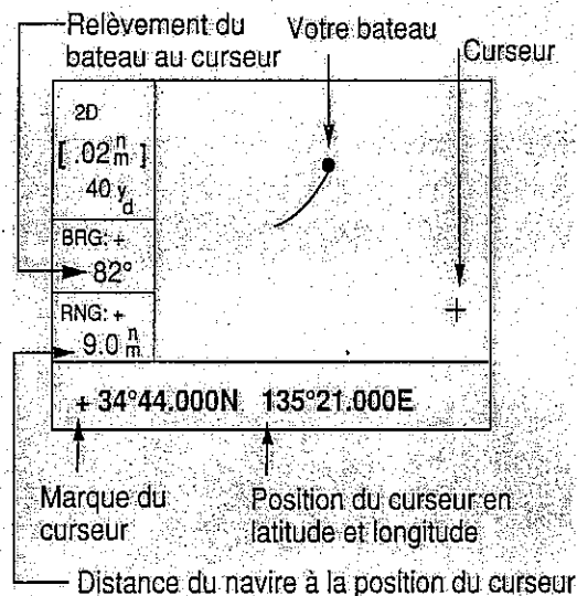
Figure 2-3 Ecran de l'affichage TRACEUR lorsque le curseur est actif.
